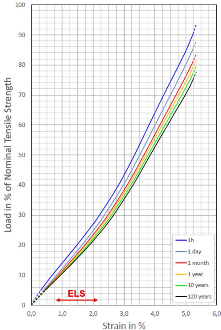
Figure 11. Domaine des déformations aux Etats Limites de Service (ELS) des géogrilles du présent projet représenté sur le graphe des isochrones des géogrilles en PVA illustrant l'évolution des déformations attendues (à court et long termes) en fonction du taux de travail des géogrilles (charge de service/traction à la rupture à court terme). Source : catalogue
