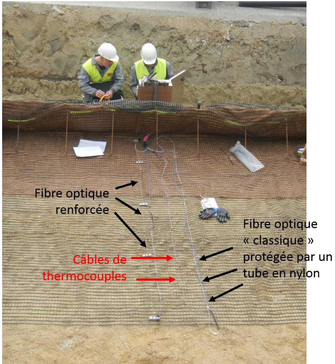
Figure 17. Installation des câbles de mesure le long de la géogrid du NIVEAU 1 pour le remblai renforcé incliné – vue 2. Source CSTC.
