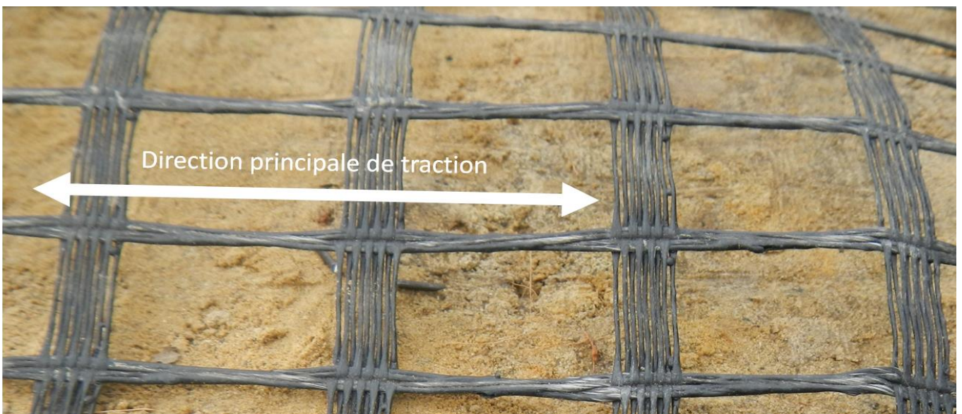
Figure 8. Géogrille
