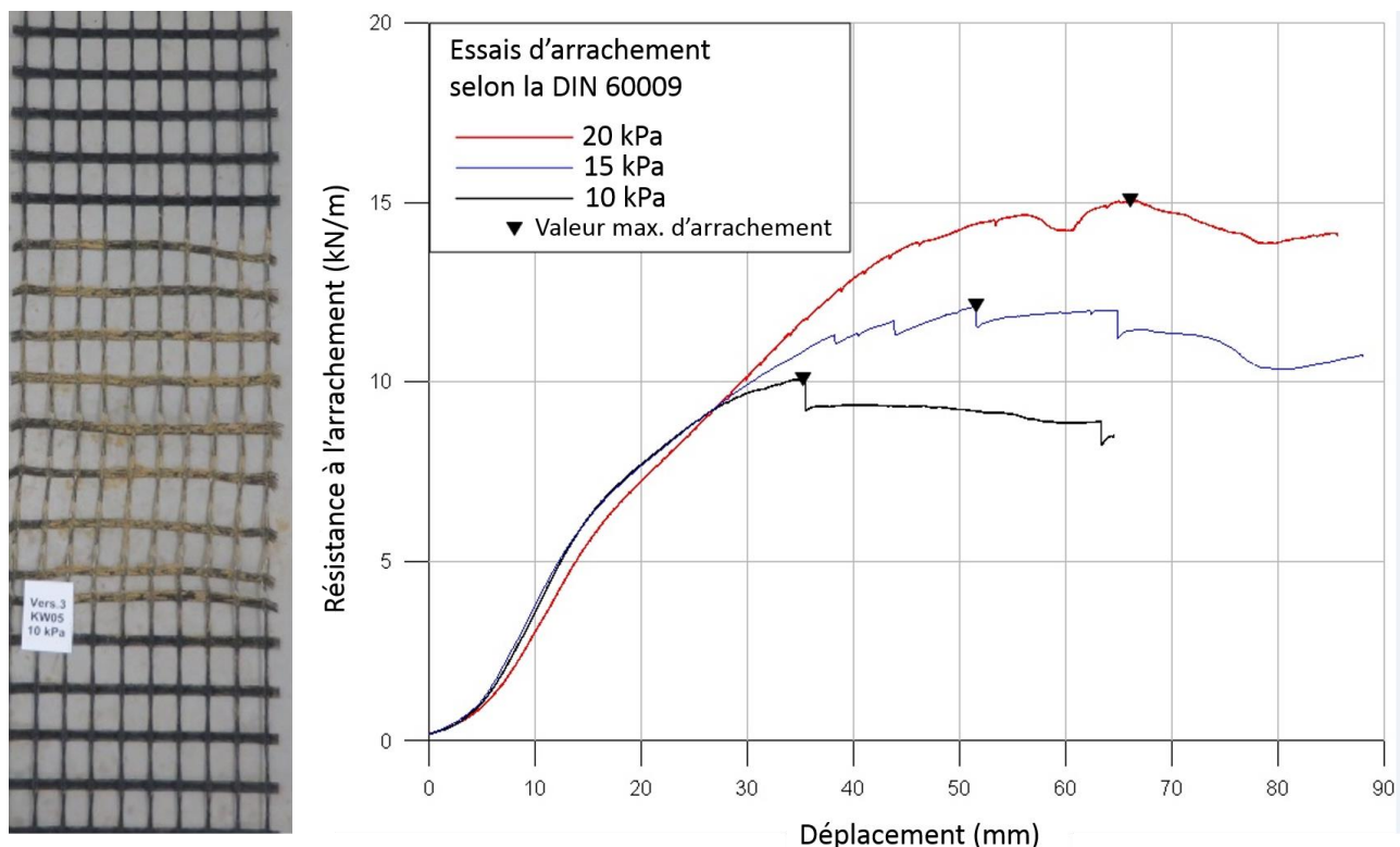
Figure 12. Résultats du test d'arrachement mené à l'interface « sol-géogrid ».
