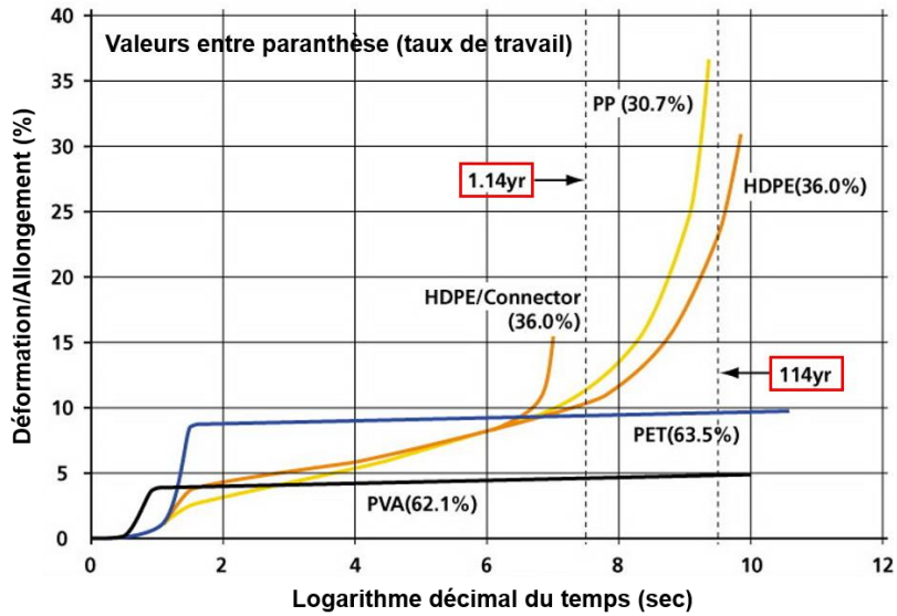
Figure 10. Comportement au fluage de différents polymères. Source : catalogue du fabricant.
